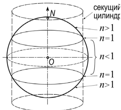
Рис.4.6. Использование секущего цилиндра
