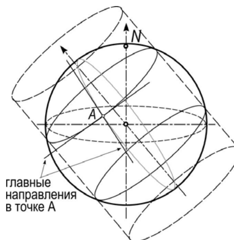
Рис.4.4. Использование косого цилиндра
