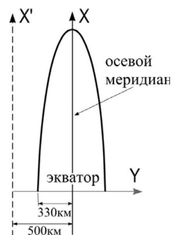
Рис.4.11. Система координат в 6^\circ -ной зоне Гаусса-Крюгера
