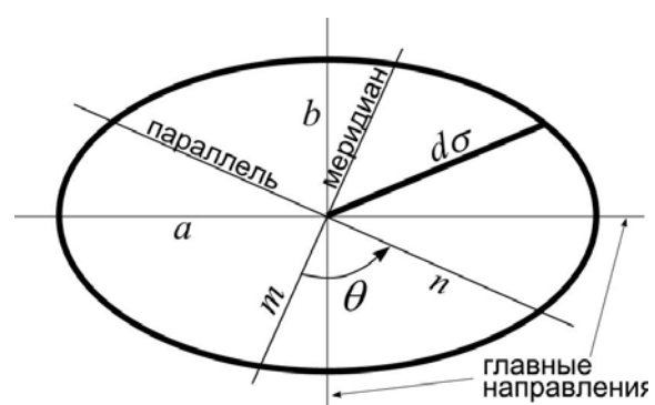
Рис.4.3. Эллипс искажений
