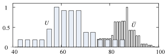
Рис. 4. \bar{U} – гистограмма-нечеткое число, равное нечеткому максимуму всех гистограмм-нечетких чисел распределения результатов ЕГЭ студентов, поступивших в 2012 году в вузы РФ на специальность «Экономика» по конкурсному набору; U – гистограмма распределения результатов ЕГЭ вуза из середины списка ранжирования
