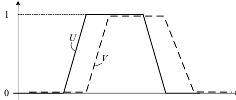
Рис. 5. Пример двух нечетких чисел, для которых r(U, V) = \Pi_U([V, +)) = 1
