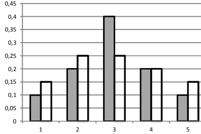
Рис. 1. Вероятностное сравнение двух гистограмм
