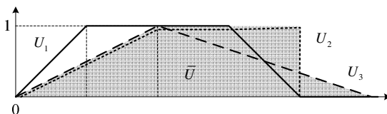
Рис. 3. Максимизация трех нечетких чисел
