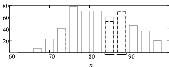
Рис. 2. Выравнивание гистограммы распределения результатов ЕГЭ студентов, поступивших в 2012 году на специальность «Экономика» по конкурсному набору в Национальный исследовательский университет «Высшая школа экономики» (г. Москва)
