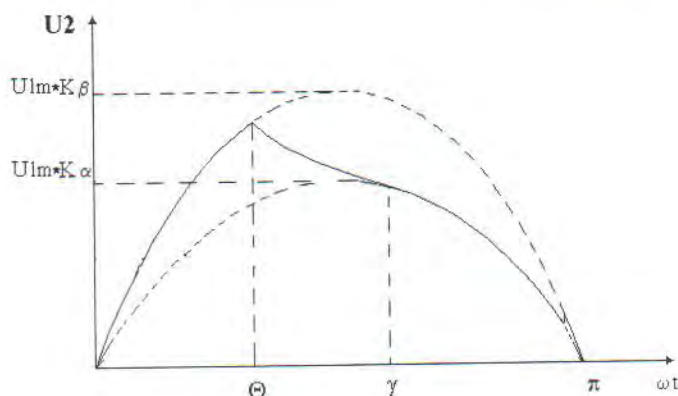
Рис. 4. Форма выходного напряжения в регуляторе с фильтрующим конденсатором
