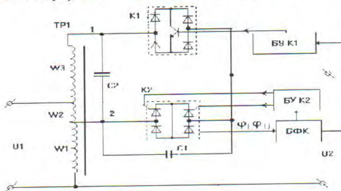
Рис. 3. Принципиальная схема регулятора переменного напряжения
