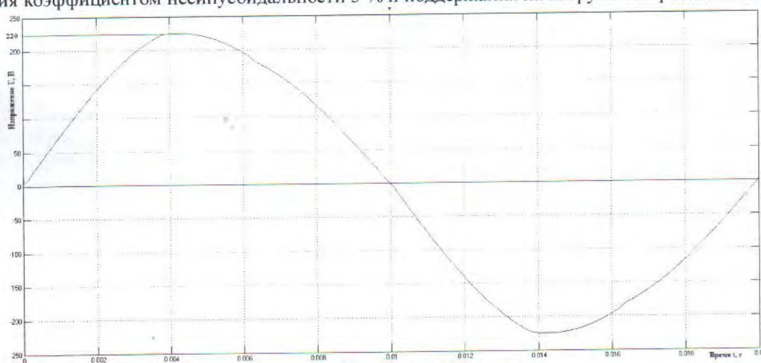
Рис. 6. Напряжение на нагрузке
