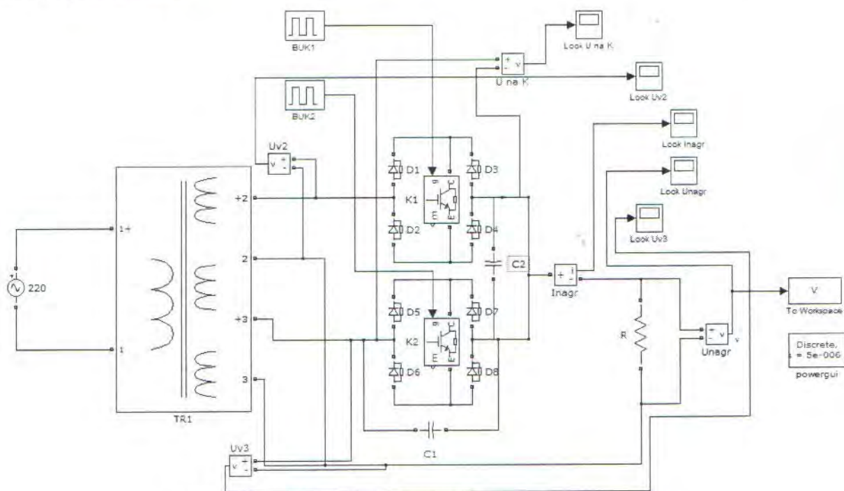
Рис. 5. Компьютерная модель стабилизации напряжения
