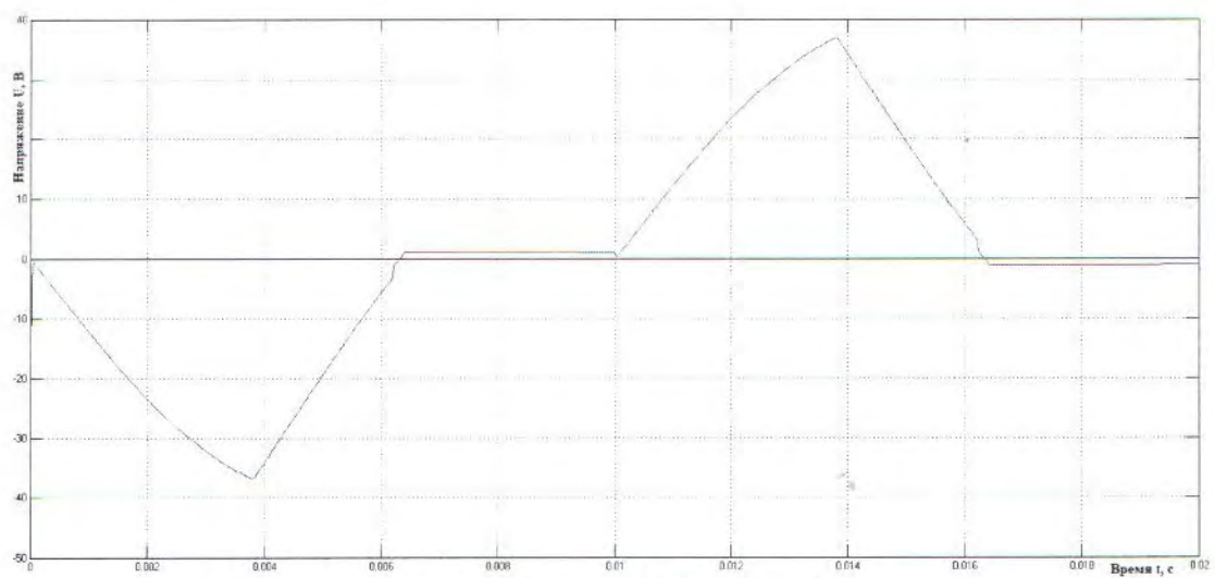
Рис. 8. Напряжение на ключе K2
