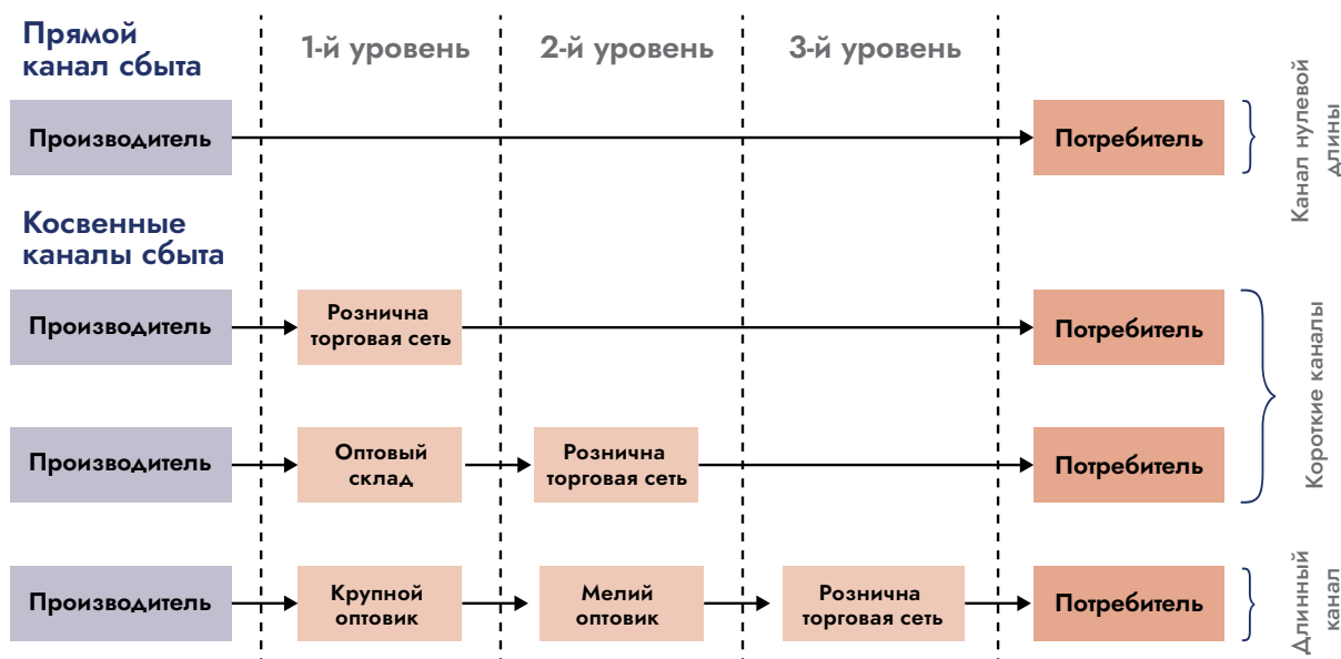
Рисунок 14. Уровни дистрибуции
