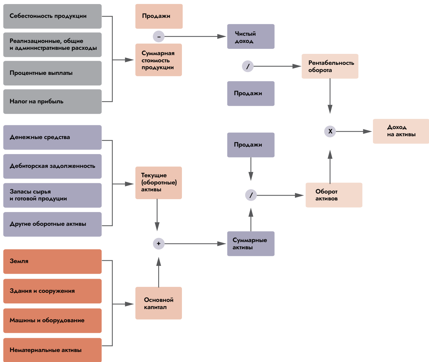
Рисунок 5. Модель прибыли
