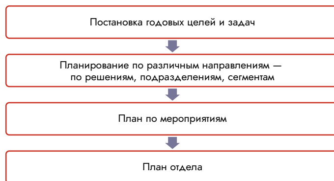
Рисунок 19. Цепочка планирования
