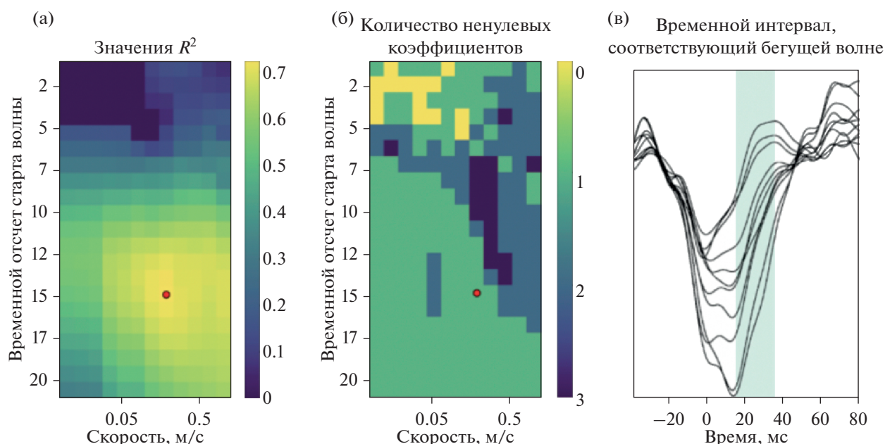
Рис. 5. Репрезентативный пример анализа одного межприступного разряда. (а) Значения R^2 , полученные для разного времени начала разряда и разных значений скорости распространения. Оптимальное решение отмечено красной точкой. (б) Соответствующие количества ненулевых коэффициентов. (в) Временные ряды МЭГ-сигналов для рассматриваемого разряда. Временной интервал, лучше всего объясненный волновой моделью, выделен цветом.
