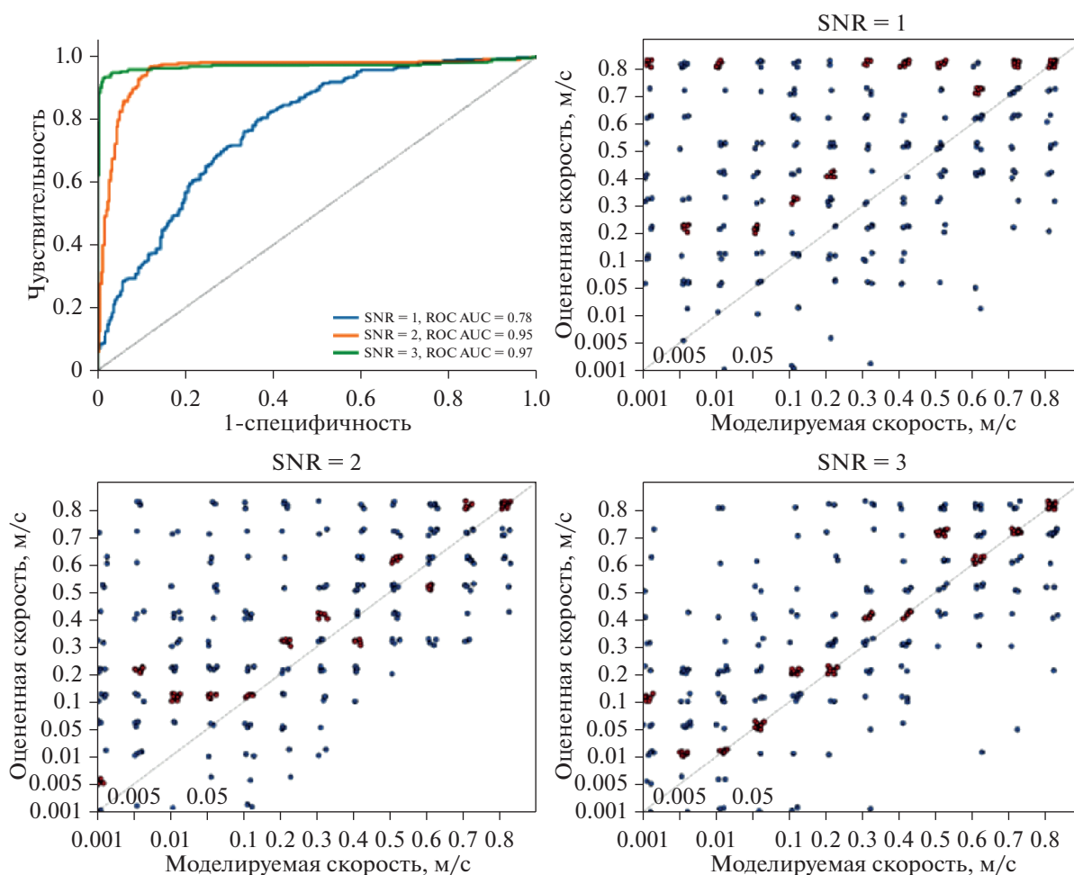
Рис. 3. Сравнение смоделированных (по оси x ) и оцененных (по оси y ) скоростей для трех уровней отношения сигнал–шум: 1, 2 и 3. Каждая точка соответствует одному испытанию методом Монте-Карло. К значениям добавляется небольшой случайный сдвиг для удобства визуализации. Для каждого значения реальной скорости определяется наиболее частое значение расчетной скорости, и соответствующие точки отображаются красным цветом.
