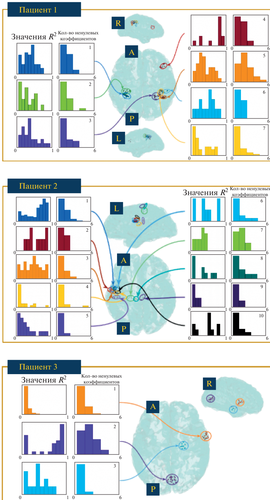
Рис. 6. Локализация эпилептических очагов, автоматически обнаруженных методом ASPIRE для трех пациентов. Для каждого кластера показано распределение метрики R^2 (качество подгонки модели) и количество направлений, используемых в оптимальном решении (простота модели).
