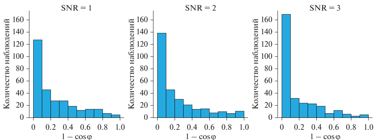
Рис. 4. Распределение ошибки детекции направления распространения 1 - \cos \phi , где \phi – угол между главным направлением истинного распространения и главным направлением оцененного распространения. Результаты показаны для 300 испытаний методом Монте-Карло и для трех уровней отношения сигнал–шум: 1, 2, 3.
