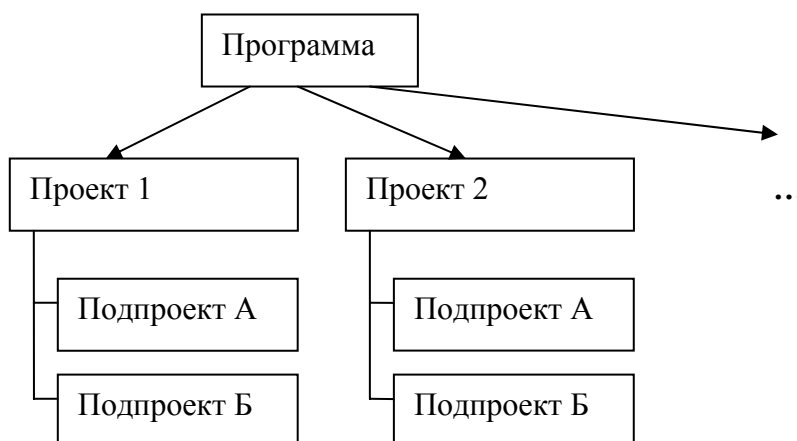
Рис. 1.1 Структура программы
