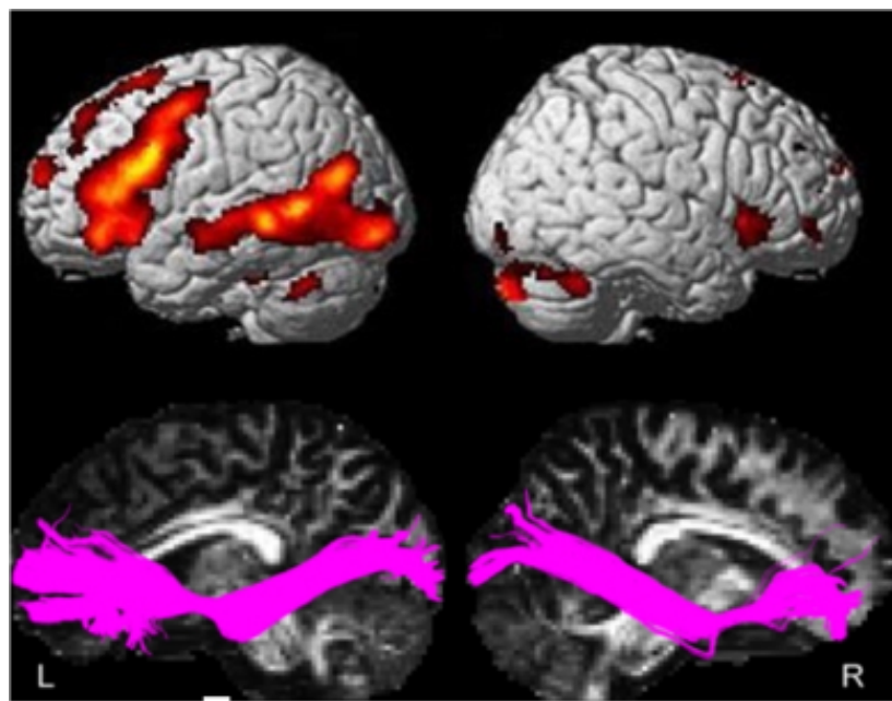
Тракт белого вещества, предсказывающий репрезентацию речи в мозге
