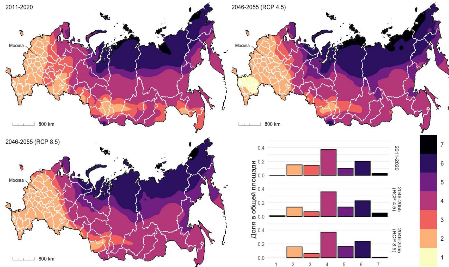
Зоны природно-климатической комфортности по данным метеонаблюдений
